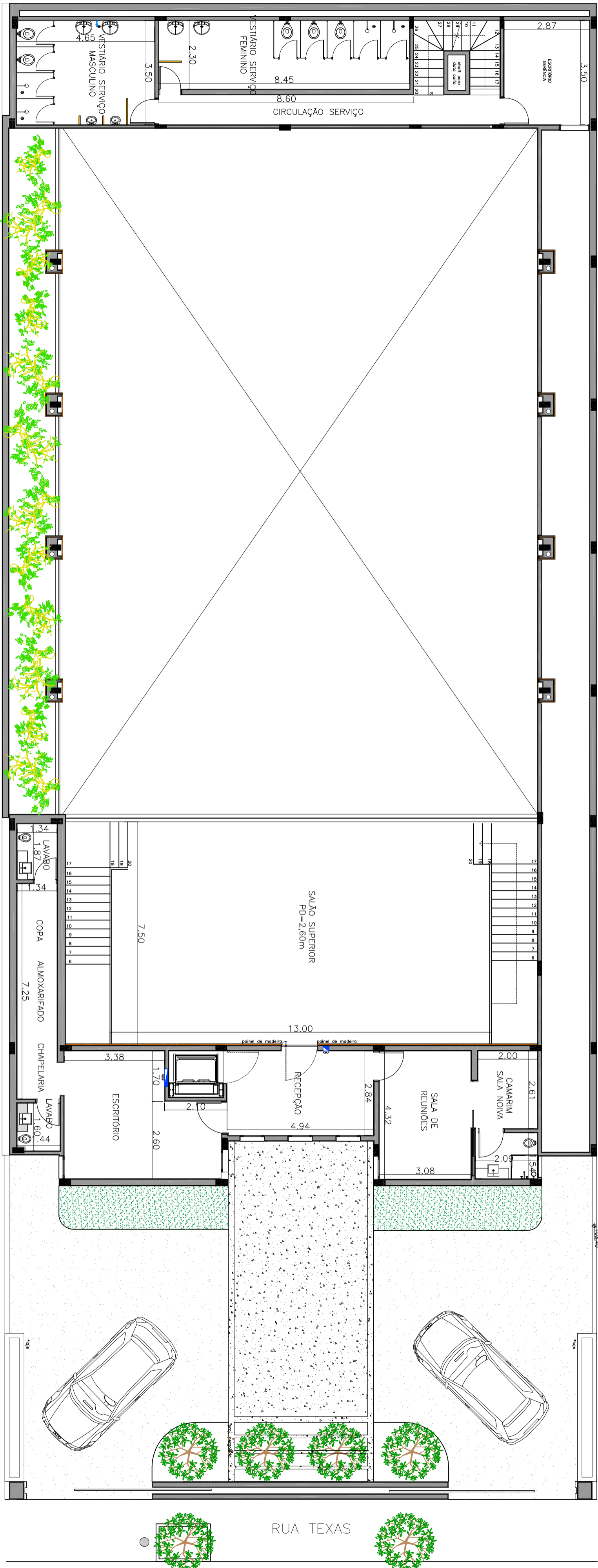
PLANTA SUPERIOR Área: 1.320 m 2 Escala: 1:50 Projeto: Indústria Sida 80 pessoas sentadas (100 operários)
